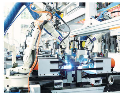
管带机核心部件——托辊智能制造生产线
