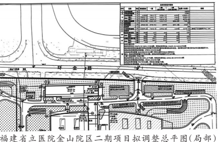
福建省立医院金山院区二期项目拟调整总平面图(局部)
